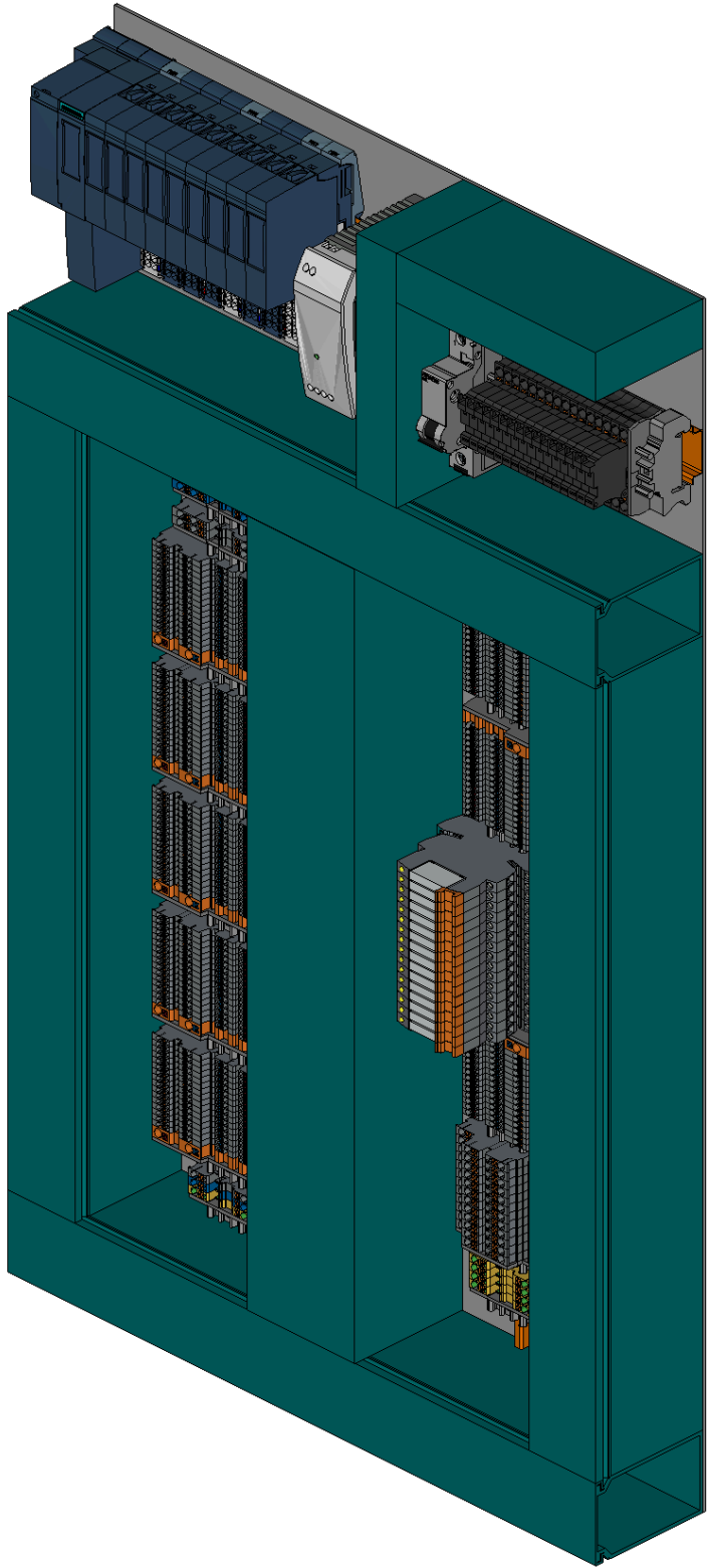
VISTA ISOMÉTRICA PLACA DE MONTAGEM
